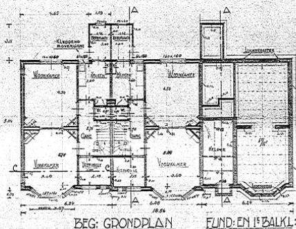
BEG. GRONDPLAN FUND. EN 1 e BALKL.
